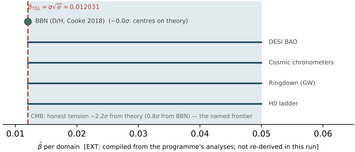
Figura 2: A convergência de \beta_{\text{TGL}} = \alpha\sqrt{e} por domínio. BBN centra na teoria ( -0,0\sigma ) como tabulada — entrada hoje RECLASSIFICADA (circular por construção; descircularizada não discrimina); os demais domínios caem na banda 0,012–0,050; a tensão CMB ( \sim 2,2\sigma ) é a fronteira honesta. [EXT: compilação das análises do programa (tgl_paper_unified.py), não re-derivada nesta rodada; a linha \beta_{\text{TGL}} é recomputada ao vivo.]
